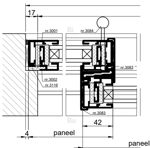
HORIZONTALE DOORSNEDE type MHS-2E
