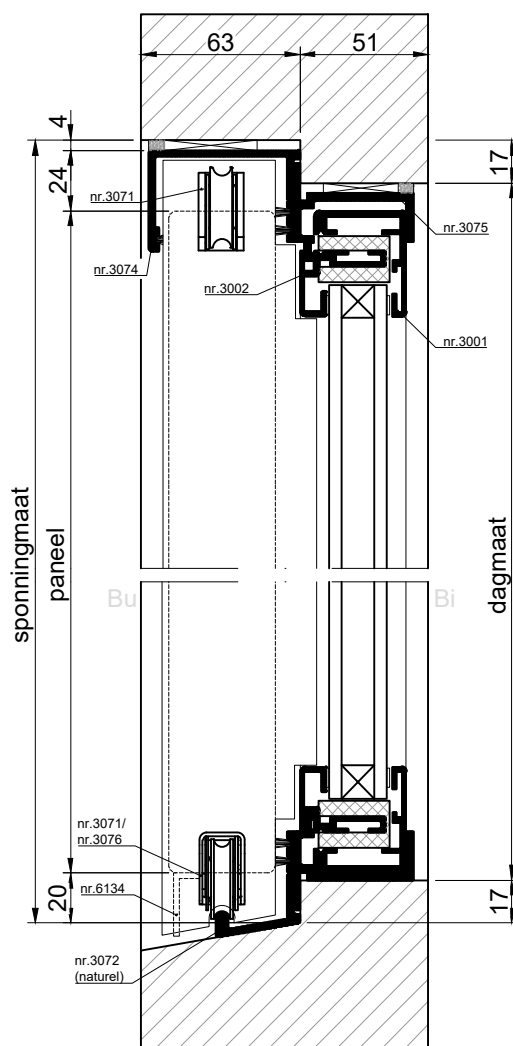
VERTICALE DOORSNEDE type MHS-2A
