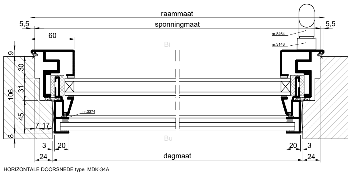
HORIZONTALE DOORSNEDE type MDK-34A
