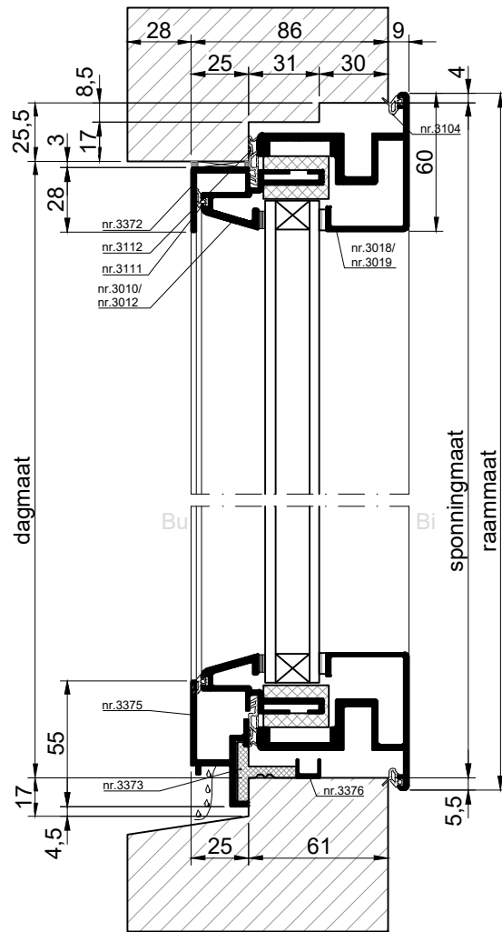
VERTICALE DOORSNEDE type MSDK-1
