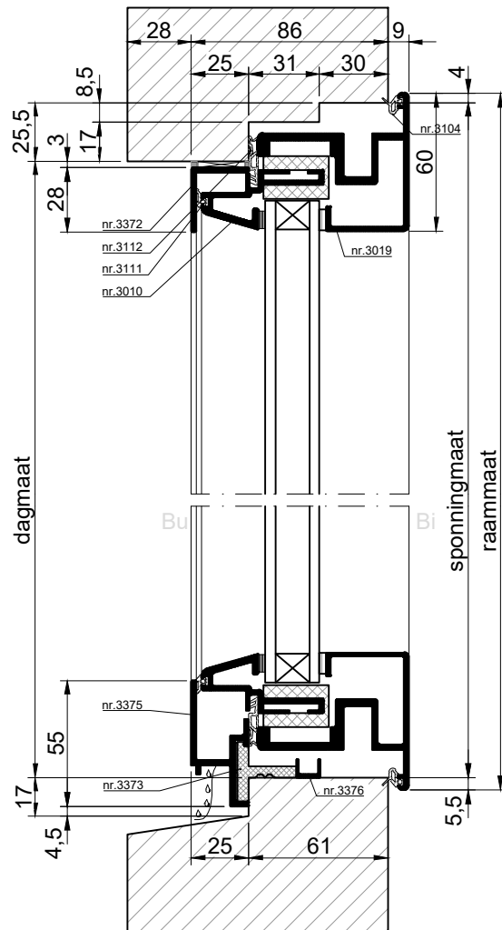
VERTICALE DOORSNEDE type MDK-30A
