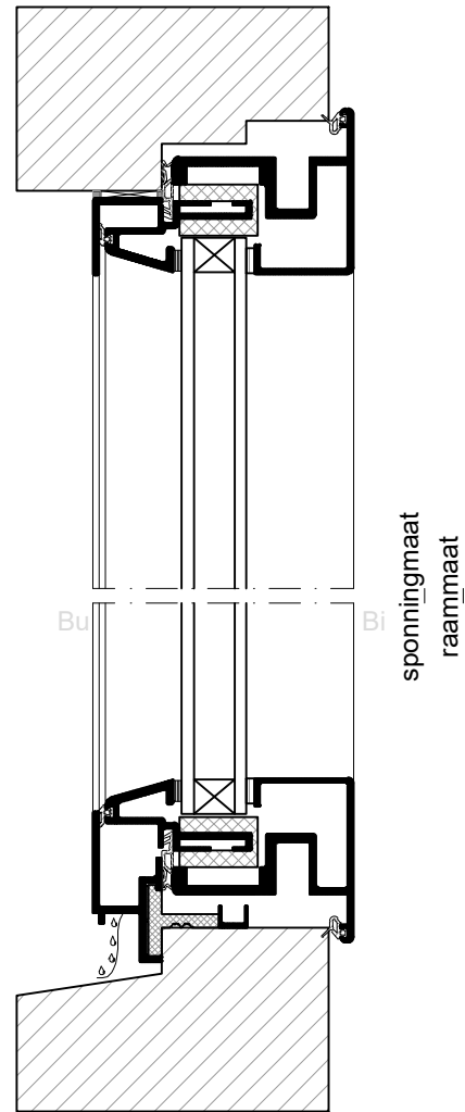
VERTICALE DOORSNEDE type MDK-30A
