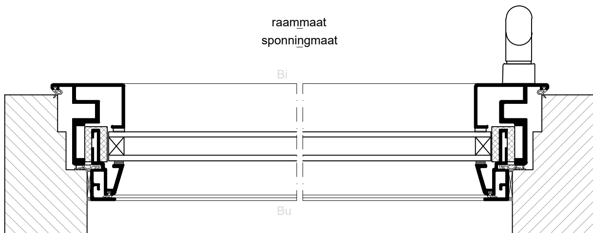
HORIZONTALE DOORSNEDE type MDK-30A
