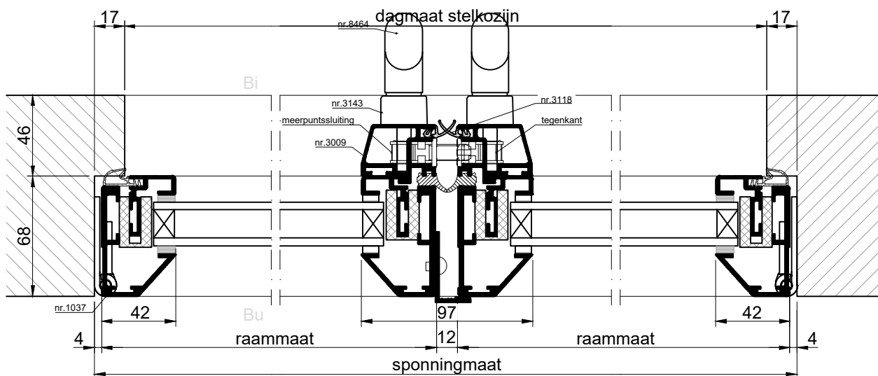
HORIZONTALE DOORSNEDE type MSU-10
