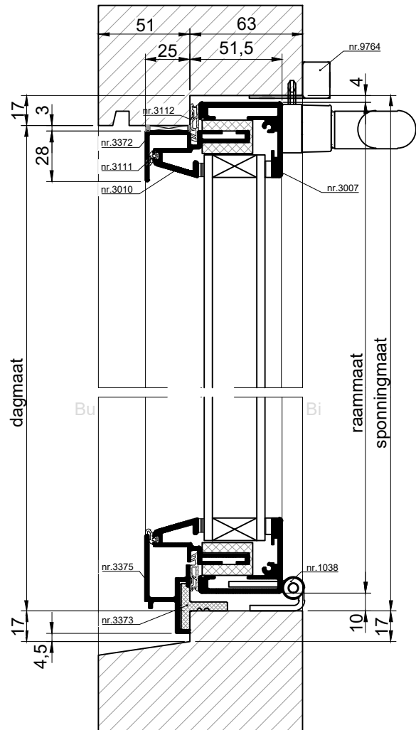
VERTICALE DOORSNEDE type MV-18
