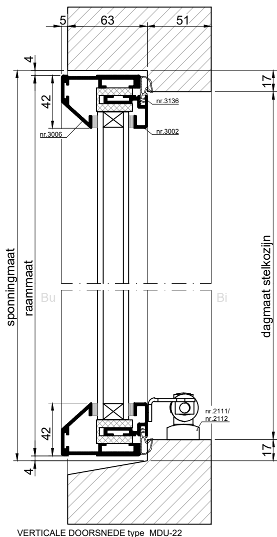
VERTICALE DOORSNEDE type MDU-22
