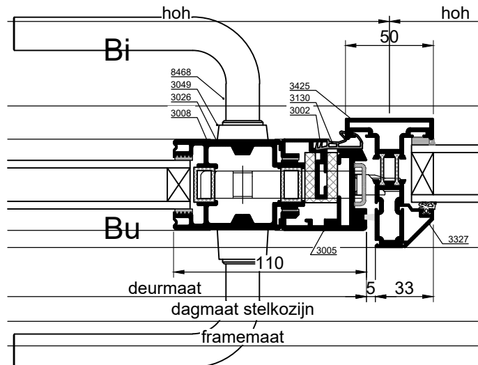
tussenstijl deur met vast deel
