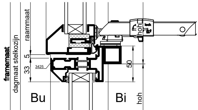
tussenstijl klepraam met vast deel
