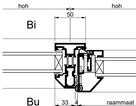
tussenstijl draairaam met vast deel
