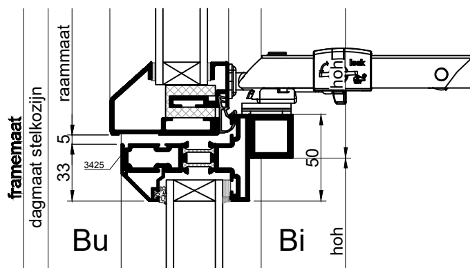
tussenstijl klepraam met vast deel
