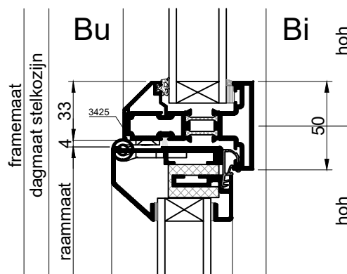
tussenstijl klepraam met vast deel
