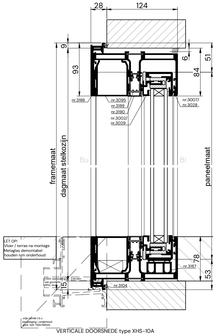
VERTICALE DOORSNEDE type XHS-10A
