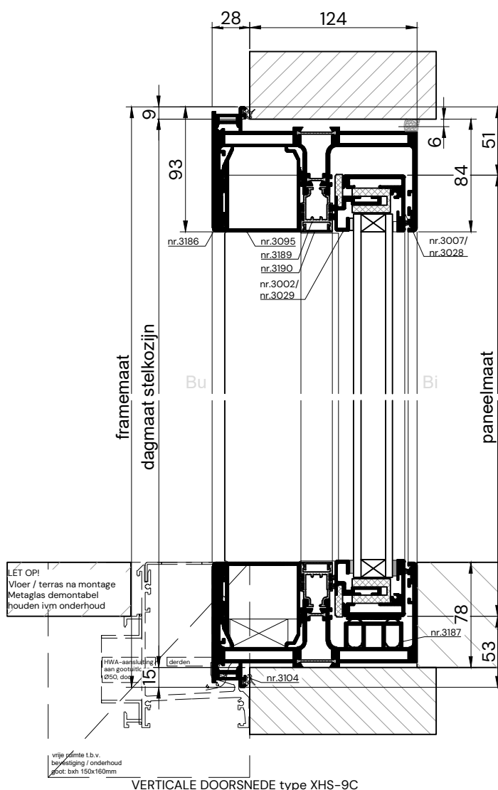
VERTICALE DOORSNEDE type XHS-9C
