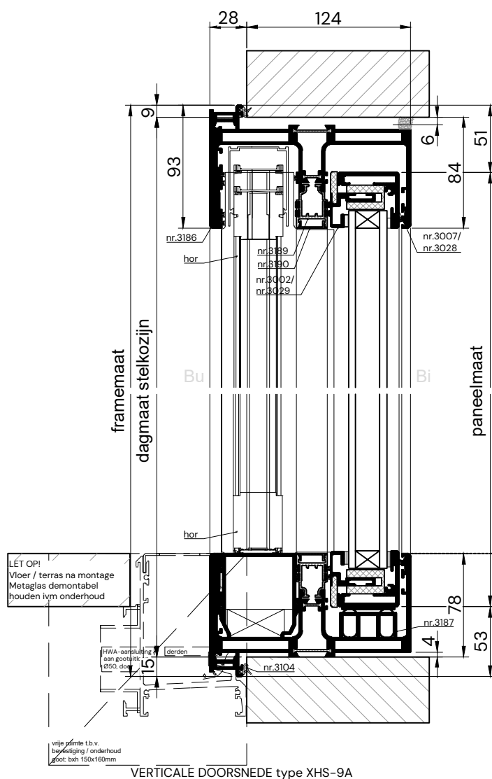
VERTICALE DOORSNEDE type XHS-9A
