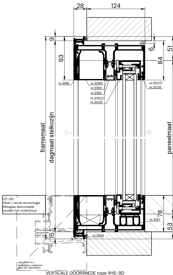
VERTICALE DOORSNEDE type XHS-9D
