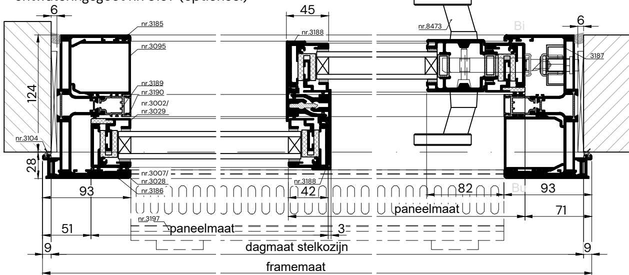
HORIZONTALE DOORSNEDE type XHS-10A
