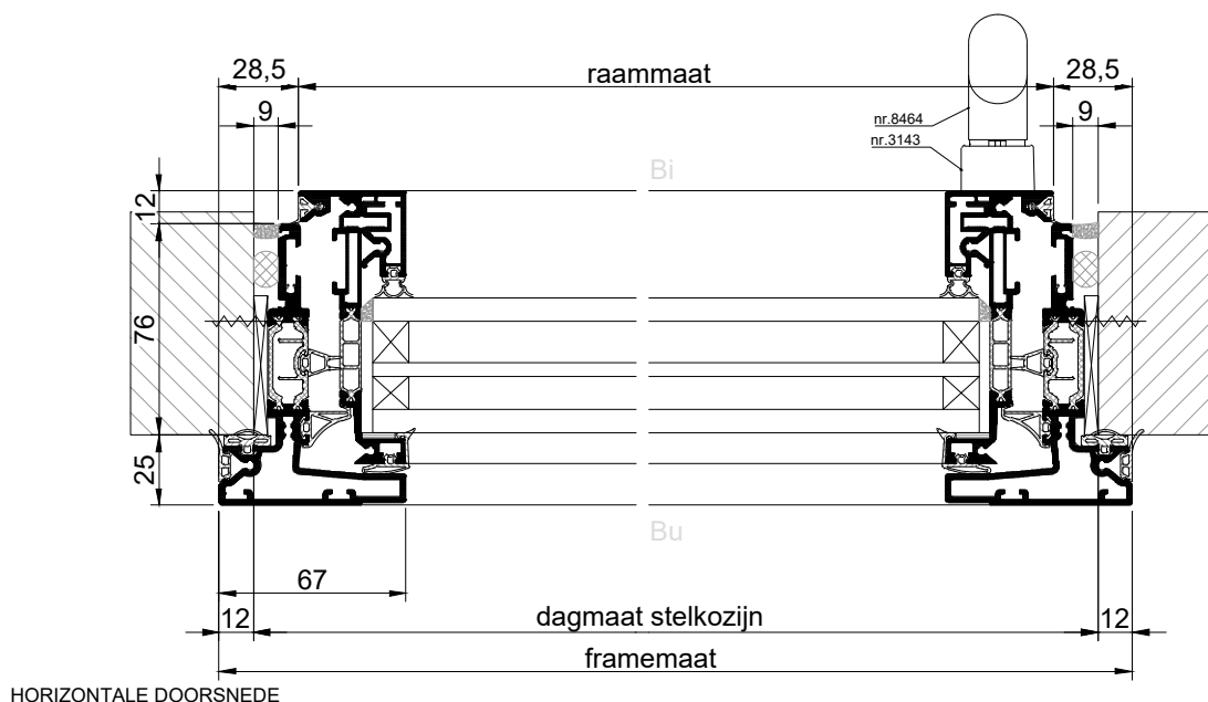
HORIZONTALE DOORSNEDE
