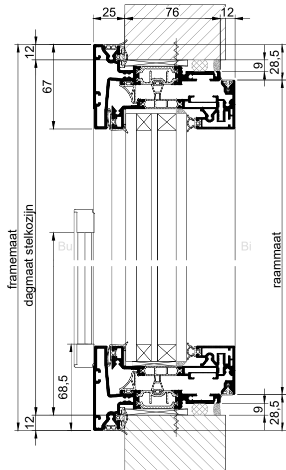
VERTICALE DOORSNEDE
