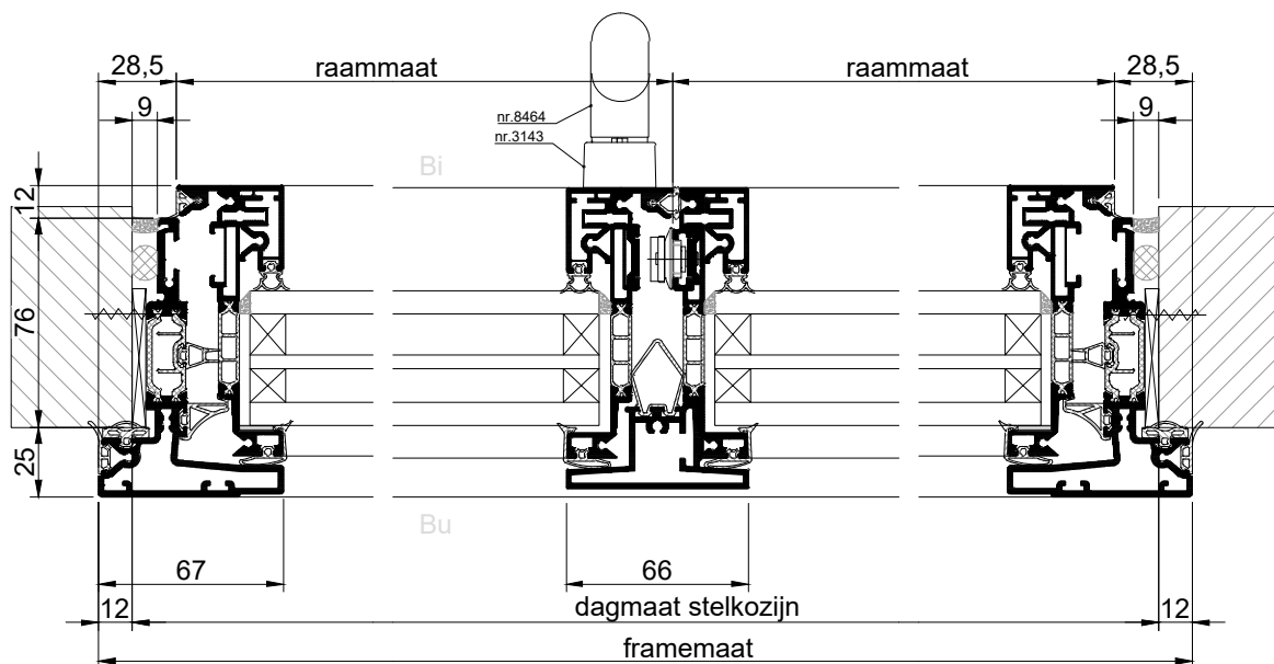
HORIZONTALE DOORSNEDE
