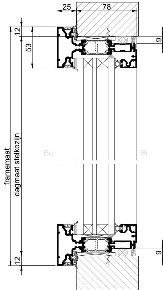
VERTICALE DOORSNEDE
