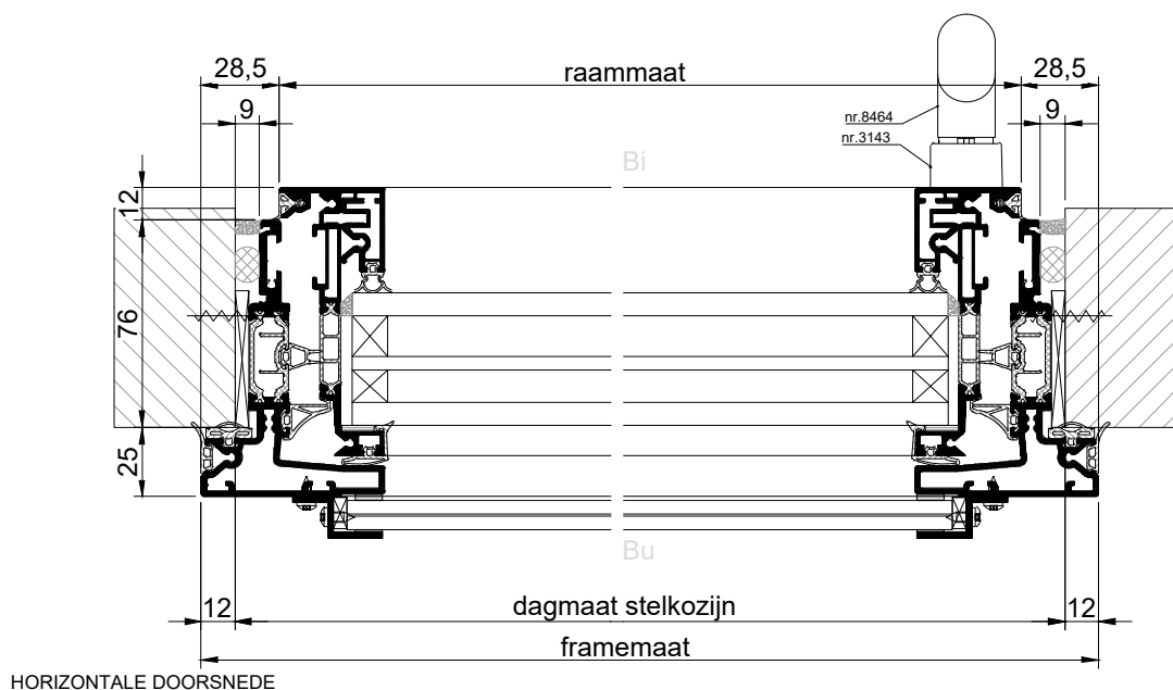
HORIZONTALE DOORSNEDE
