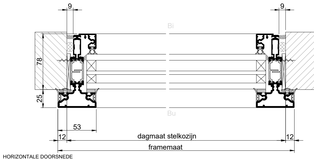
HORIZONTALE DOORSNEDE
